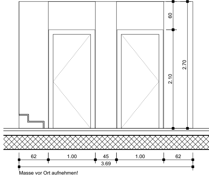
Ansicht A
