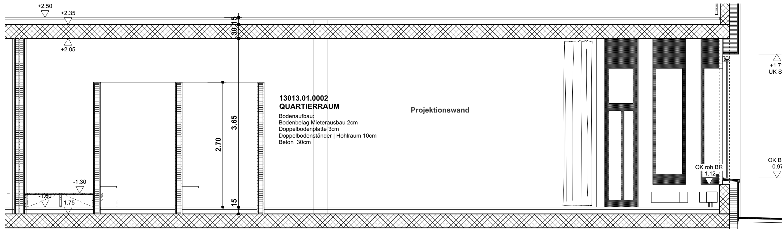
Schnitt BB
