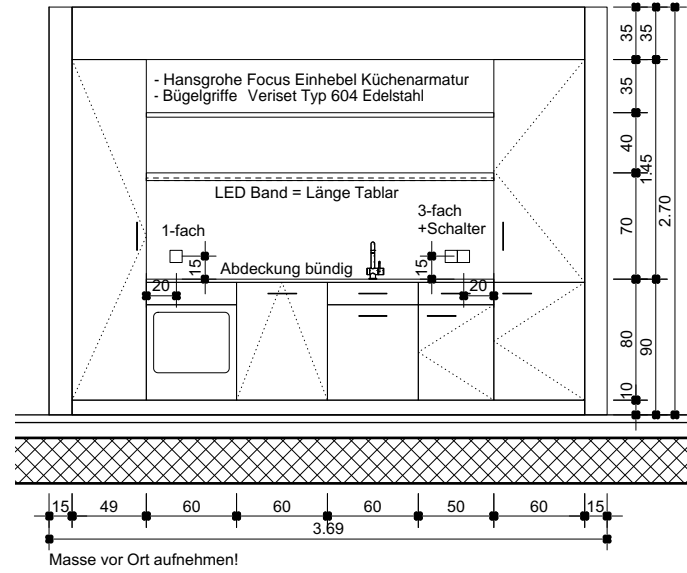
Ansicht C
