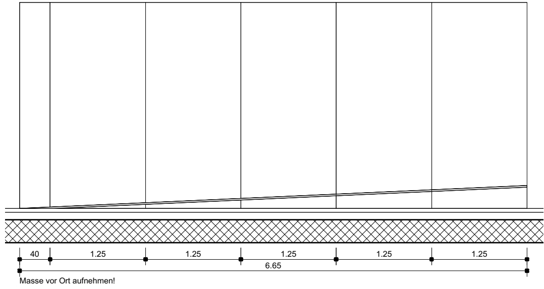
Ansicht D
