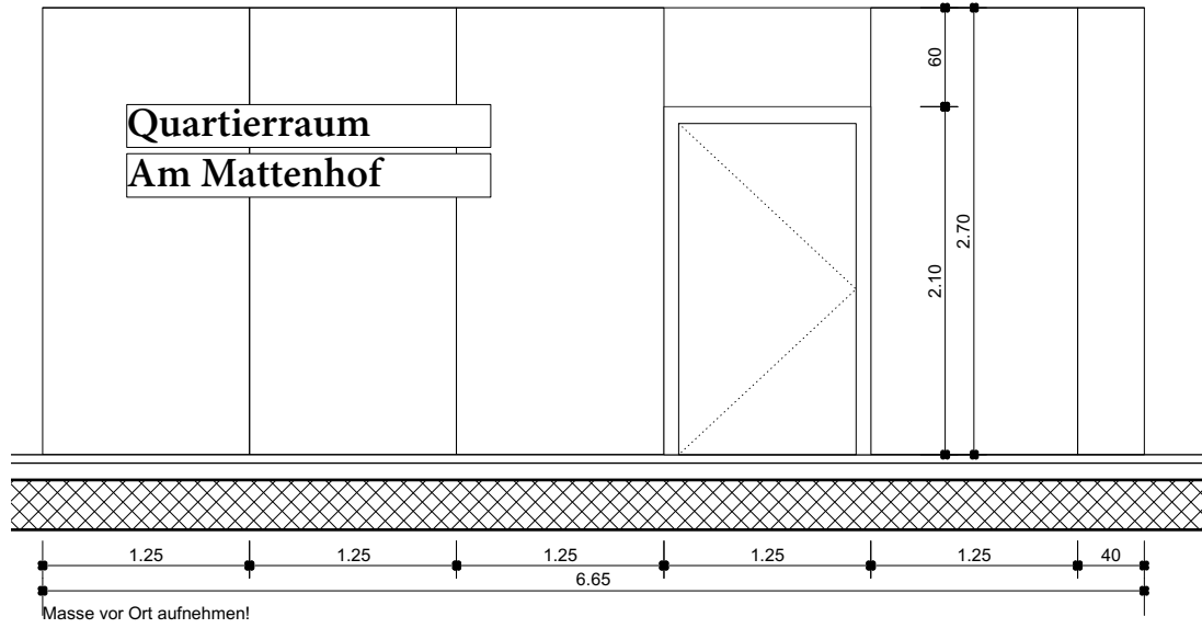
Ansicht B
