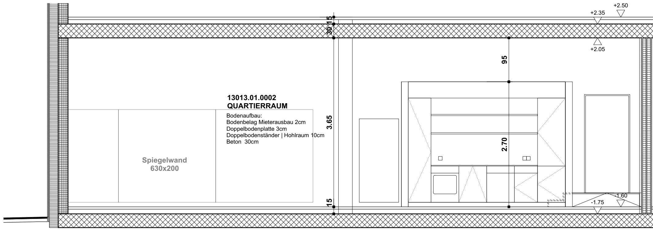
Schnitt AA
